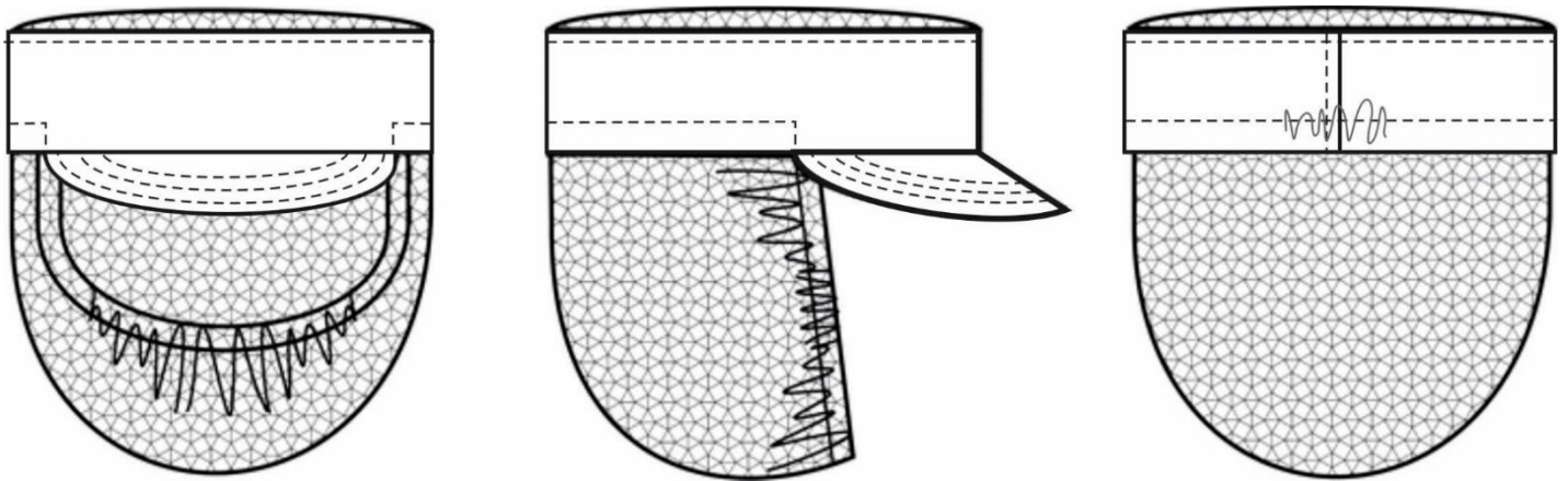
Рис.1. Эскиз Кепи универсальная с сеткой ХАССП (тк.ТиСи), белый, вид спереди, сбоку и сзади.
