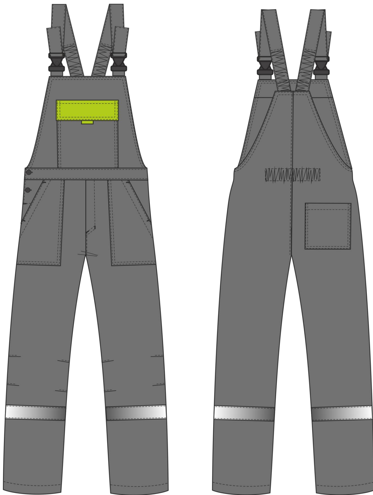
Рис.4. Костюм Фаворит-2 СОП (тк.Смесовая,210) п/к, т.серый/лимонный, Полукомбинезон вид спереди и сзади.
