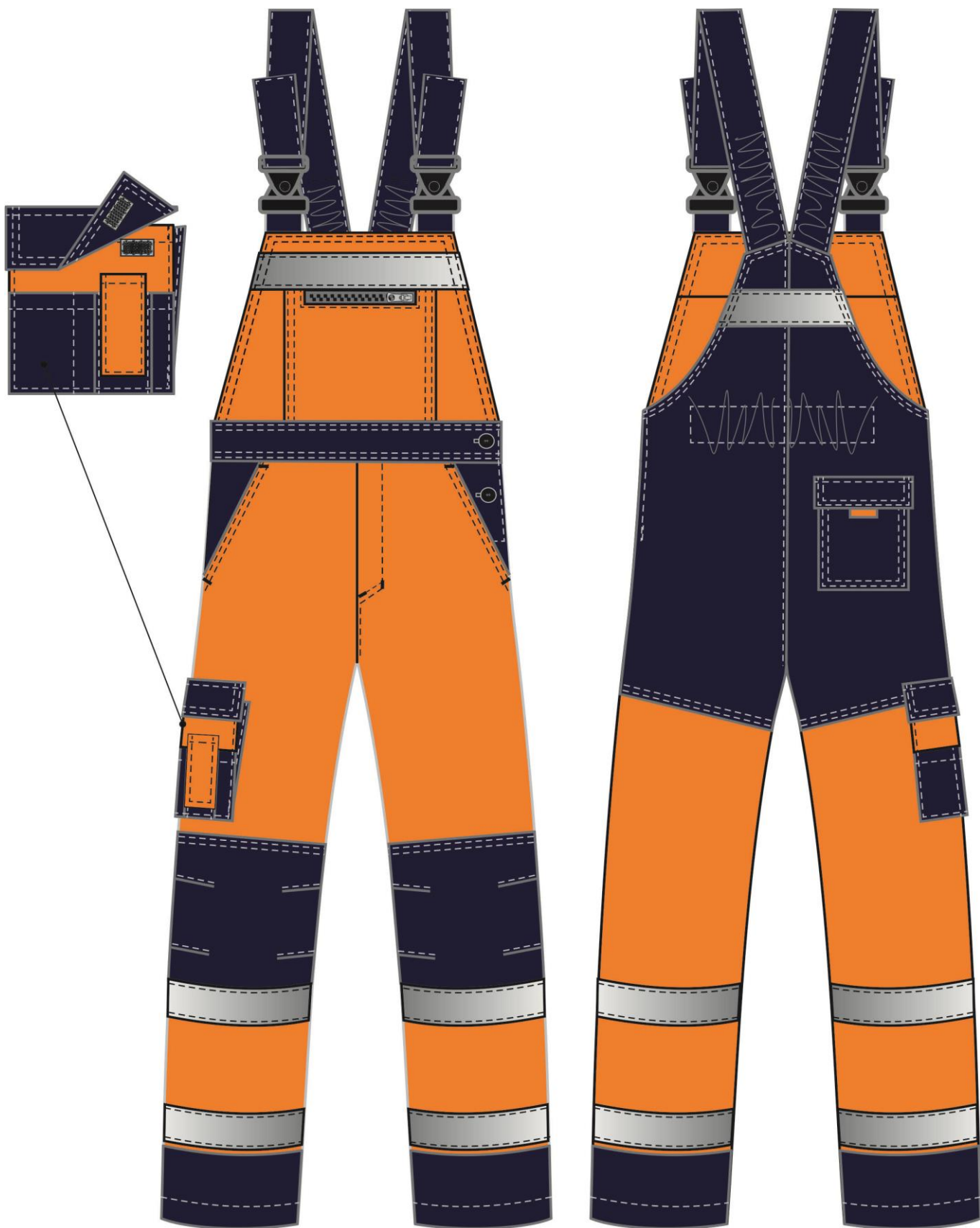
Рис.6. Эскиз Костюм дорожник Сигнал-2 (тк.Балтекс,210) п/к, оранжевый/т.синий Полукомбинезон, вид спереди и сзади.
